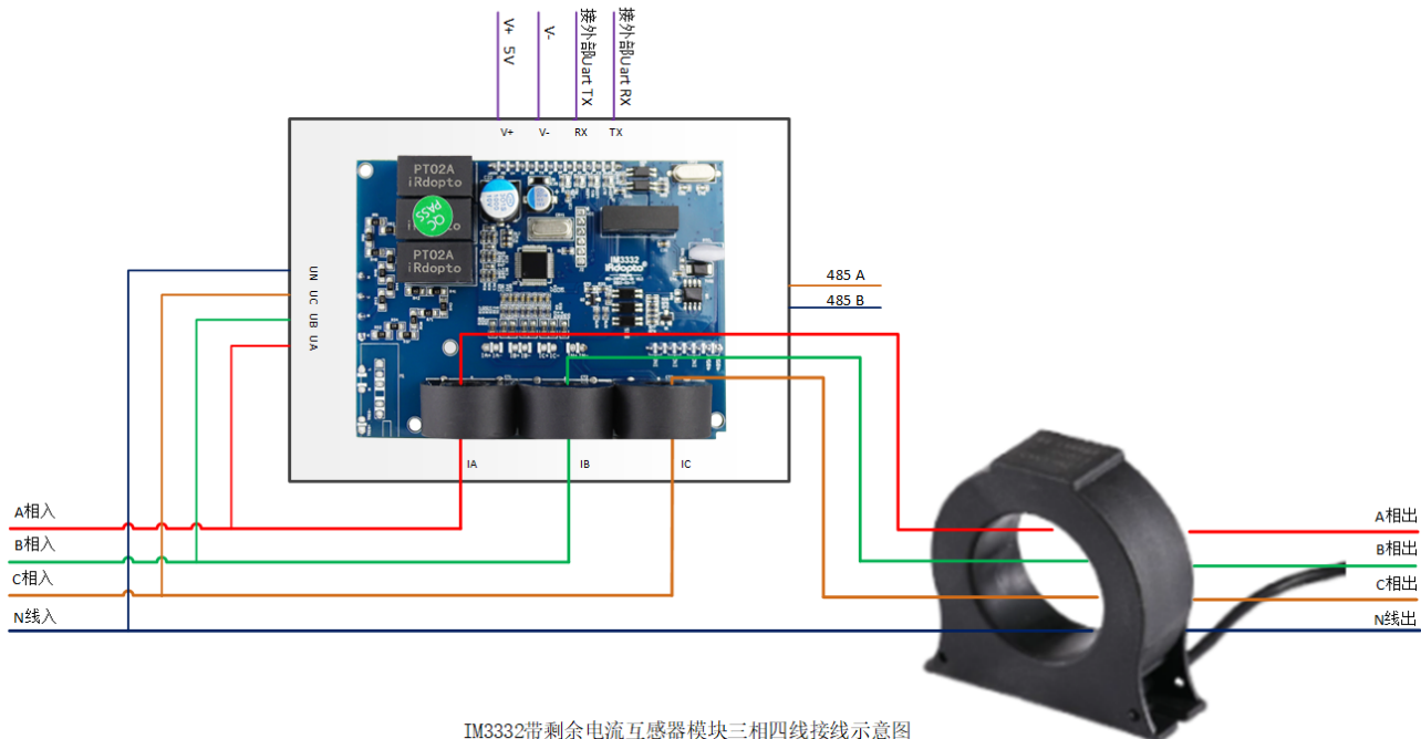
IM3332带剩余电流互感器模块三相四线接线示意图
