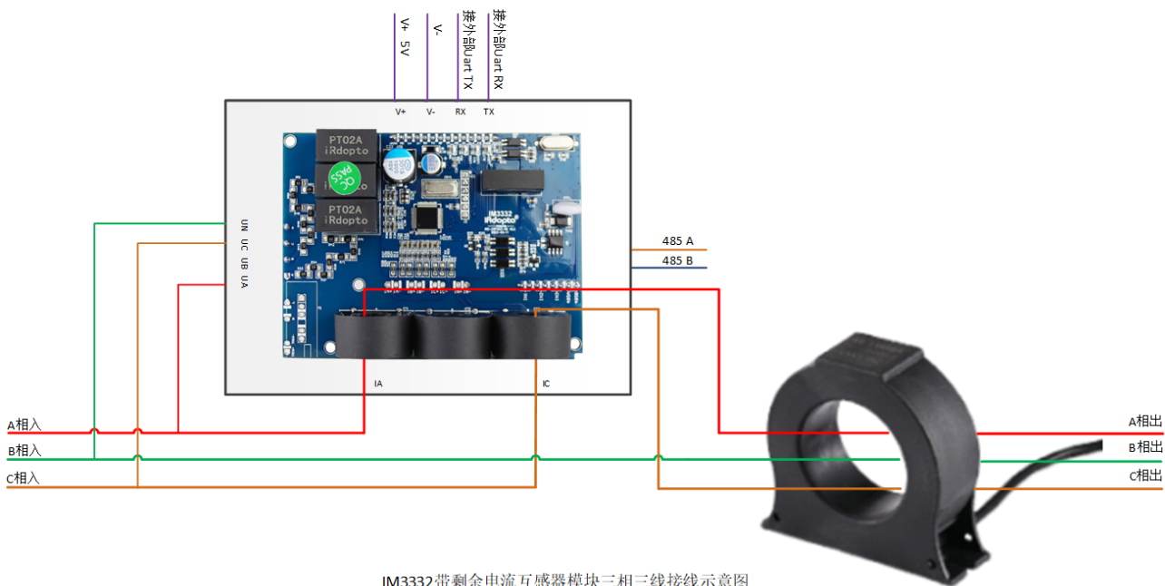
IM3332带剩余电流互感器模块三相三线接线示意图
