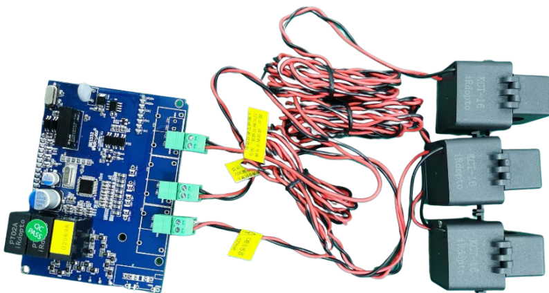
IM3332 外置开口互感器产品图 (电流支持 50A/150A/250A/500A)
